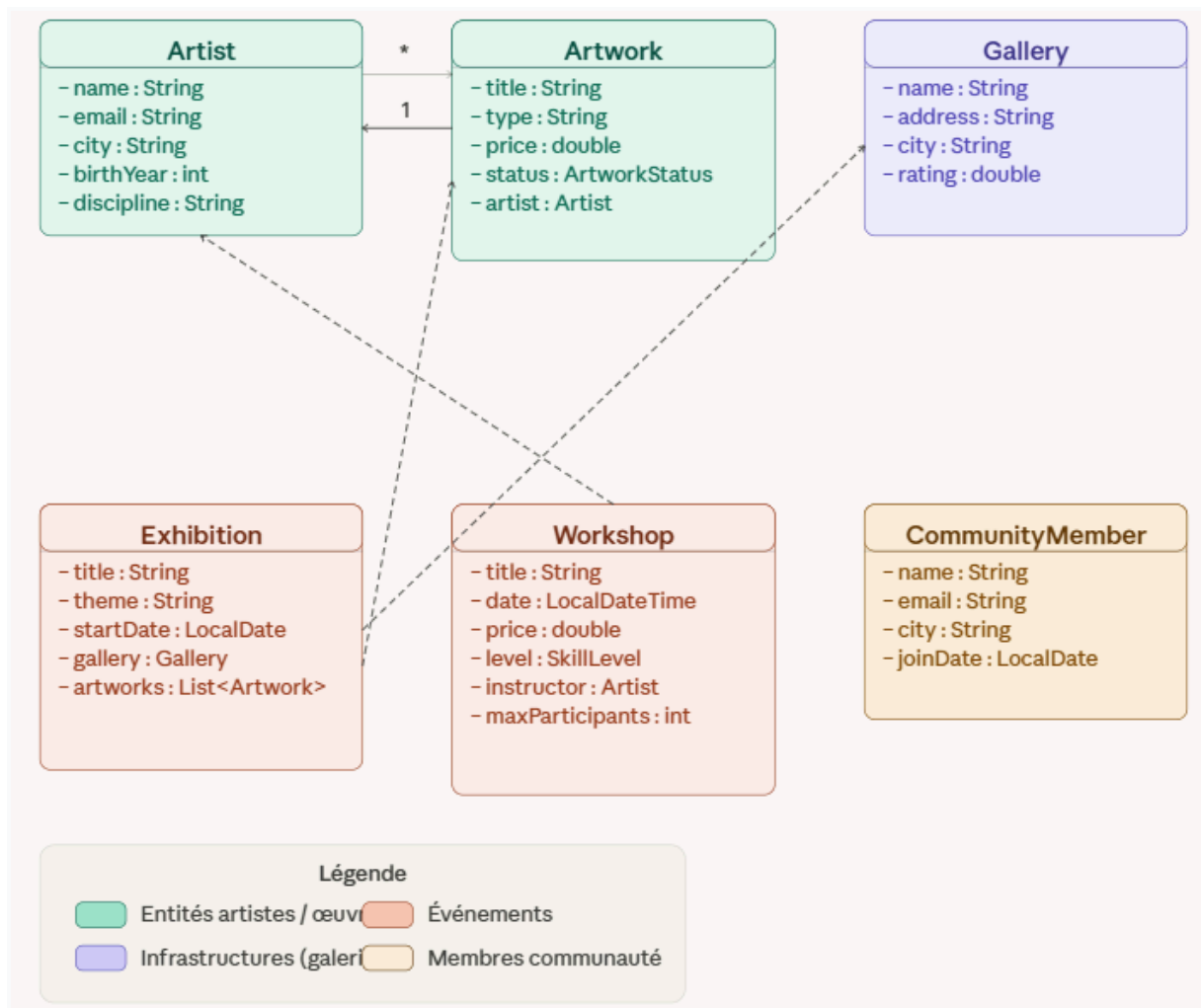
Diagramme de classes simplifié du modèle ArtConnect (Relations bidirectionnelles: Artist ↔ Artwork)
